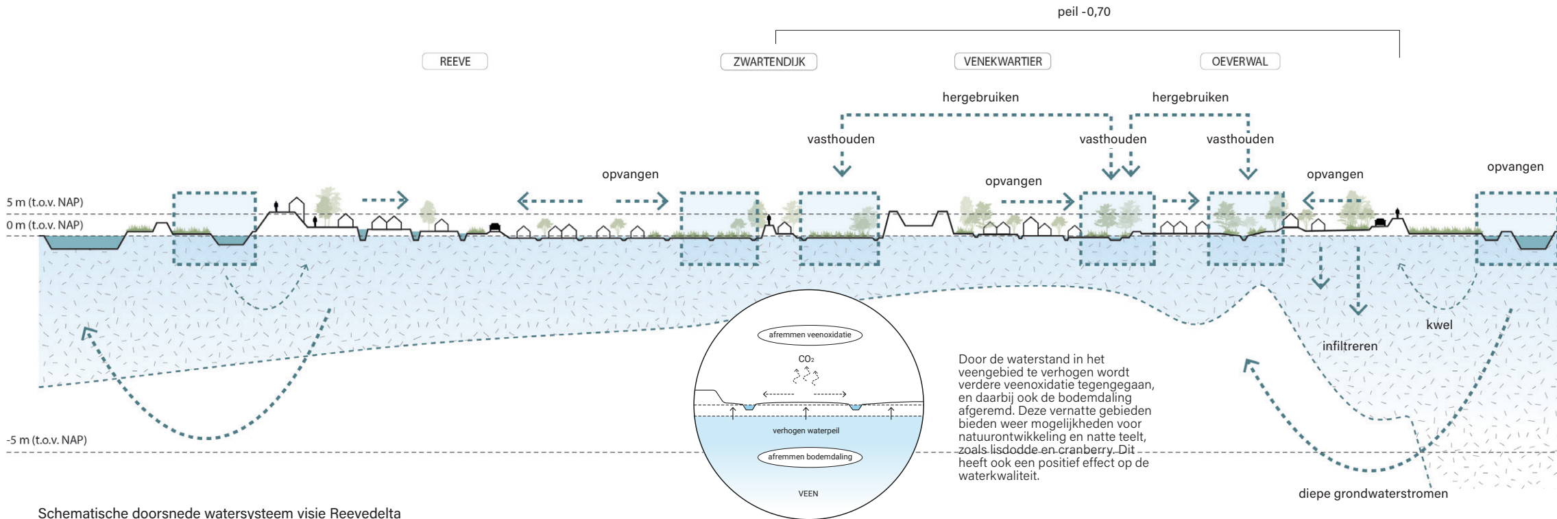
Schematische doorsnede watersysteem visie Reevedelta
