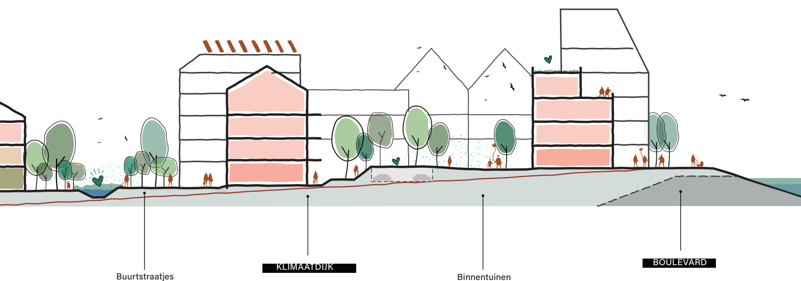
Bouwen op een brede klimaatdijk
