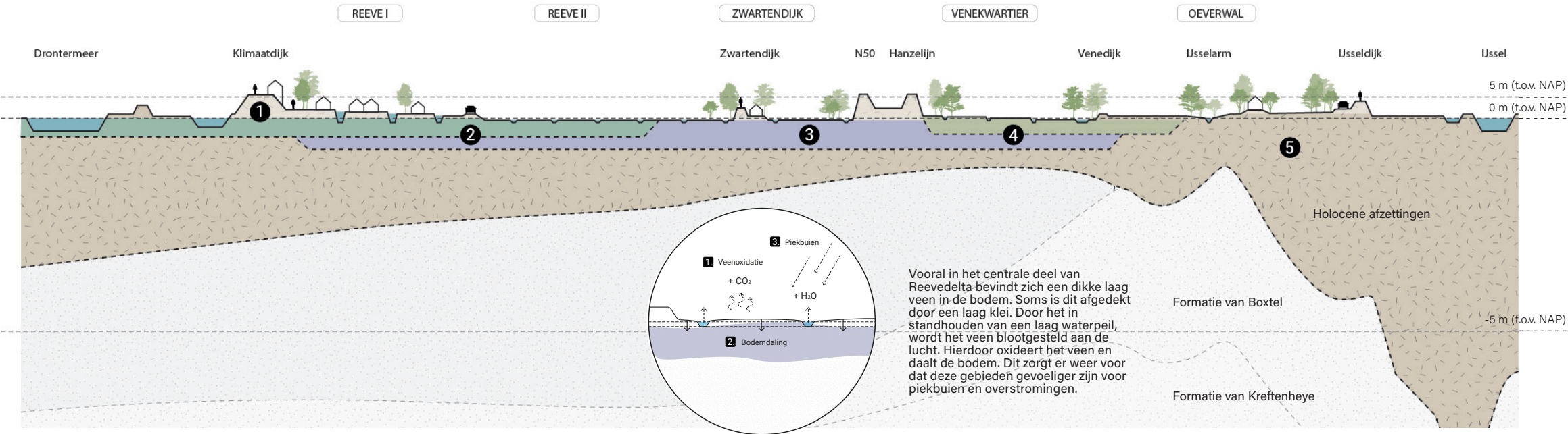
Schematische doorsnee Reevedelta (Bron: Dinoloket)
